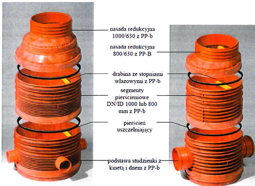
Rys.2 Studzienka PRO 1000
