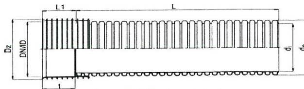
Rysunek 2. Wymiary rur K-2
